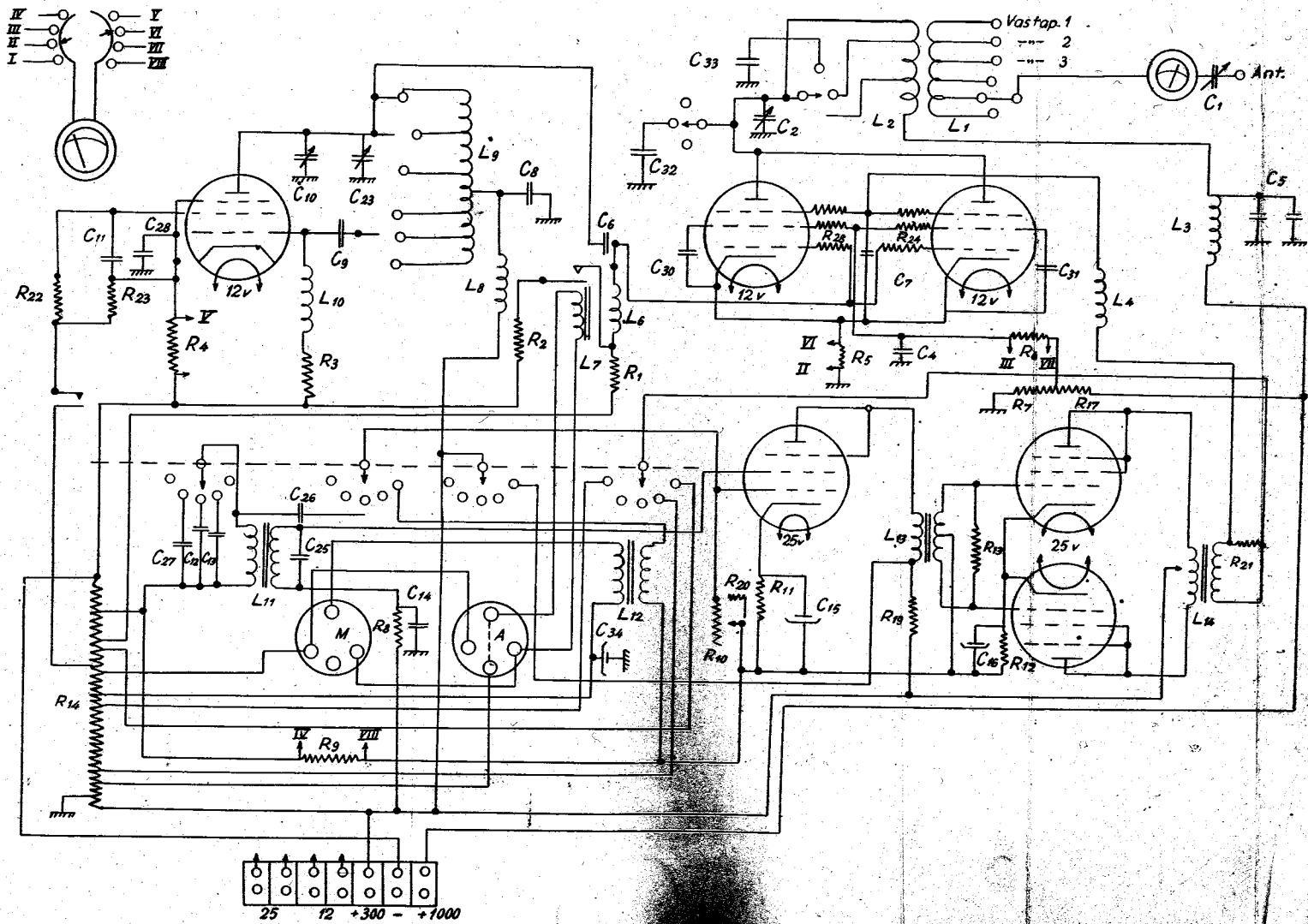
P-12-4: lähettimen kytkentäkaavio.
