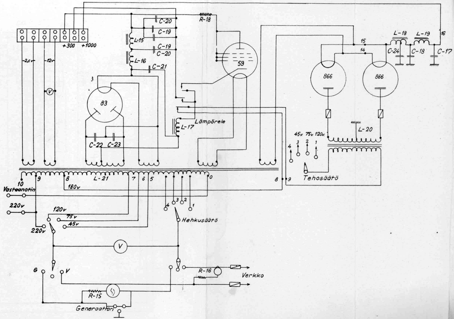
P-12-4: lähettimen virranjako- ja tasasuuntauskytkentäkaaviot.
